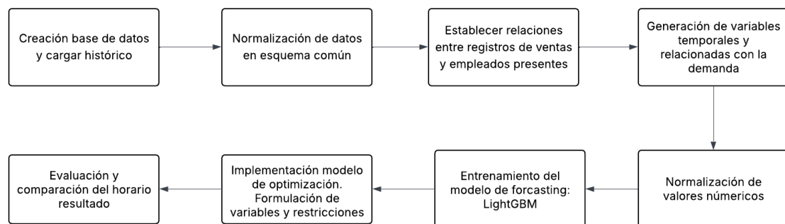
Ilustración 4: Diagrama de flujos - Módulo 2: Generador de horarios.
